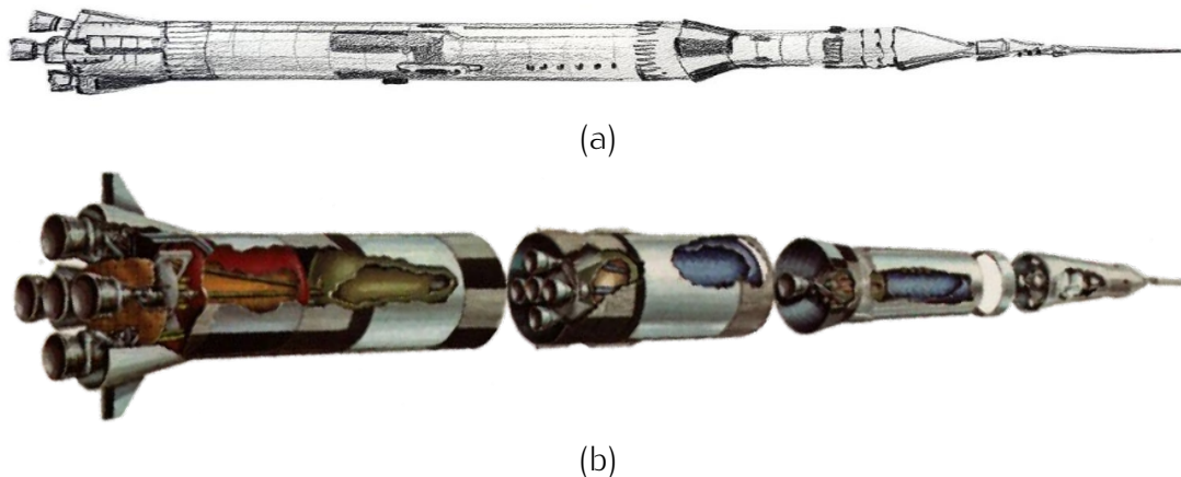
Figura 3.11: Concepção artística do foguete Saturno V completo (a) e decomposto em estágios (b).
