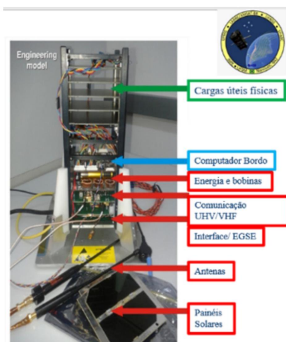
Figura 5.2: Estrutura padrão CubeSat-2U do NanosatC-BR2.
