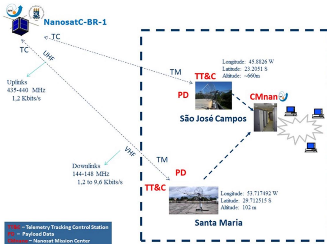
Figura 5.4: Canais de comunicação para operação da missão NanosatC-BR1.
