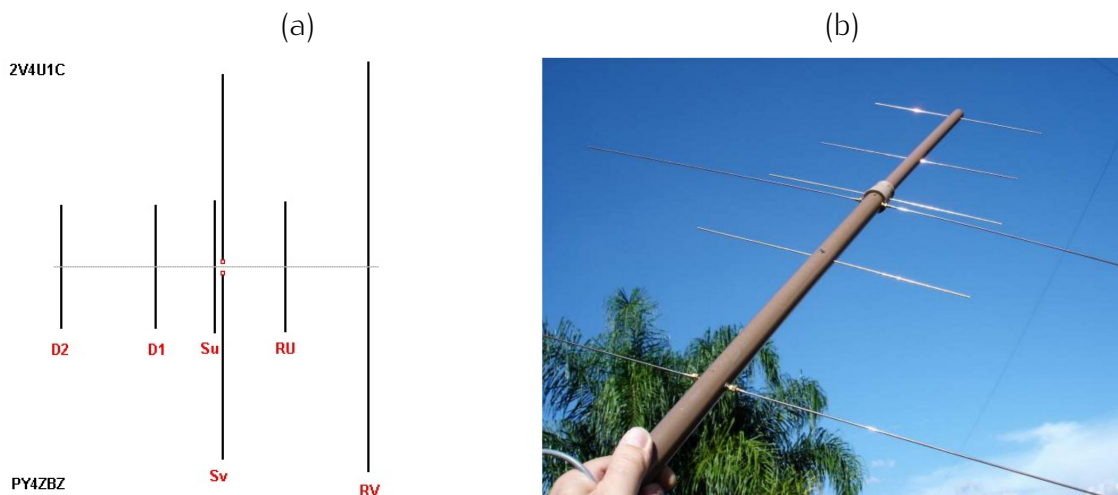
Figura 4.8: (a) Projeto de antena artesanal. (b) Antena de construção artesanal.
