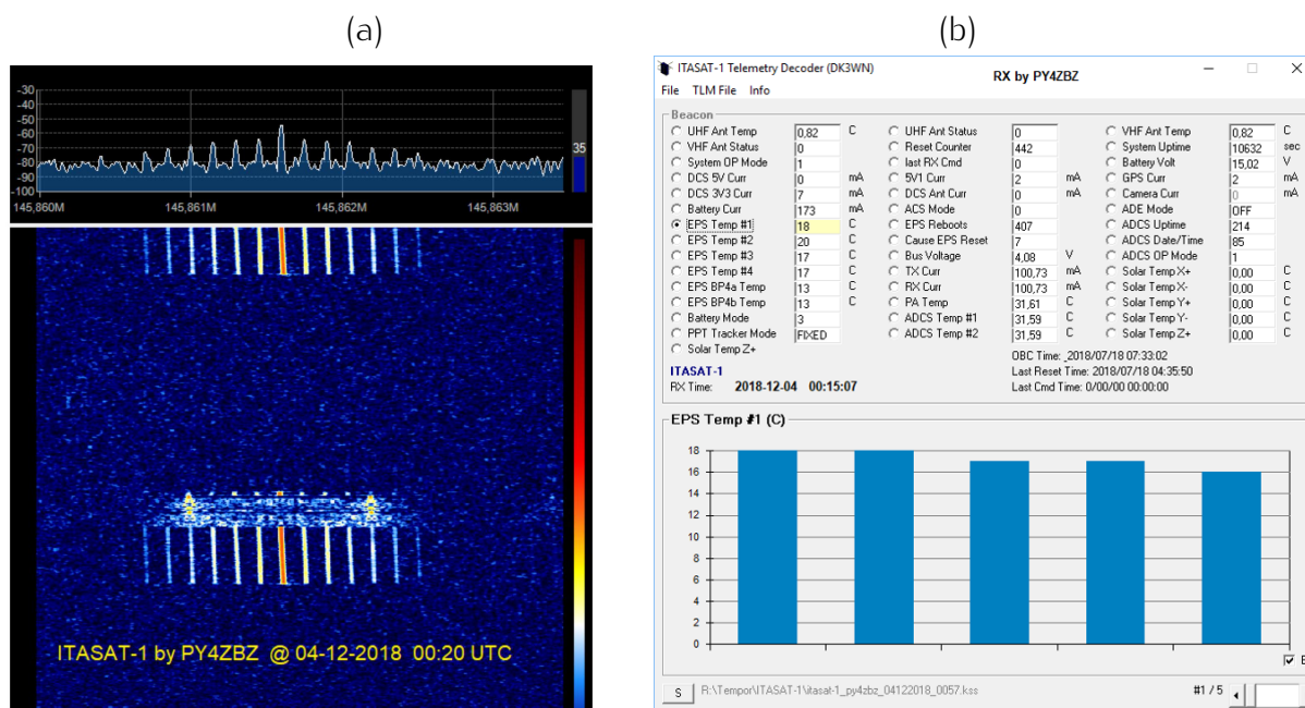
Figura 4.9: (a) Recepção e (b) Decodificação dos sinais de telemetria do satélite ITASAT-1 utilizando uma antena simples.
