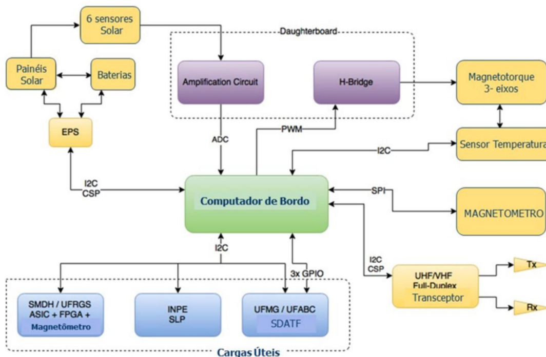
Figura 5.5: Interfaces de comunicação do C&DH do NanosatC-BR2 com os demais subsistemas da plataforma e cargas úteis físicas.
