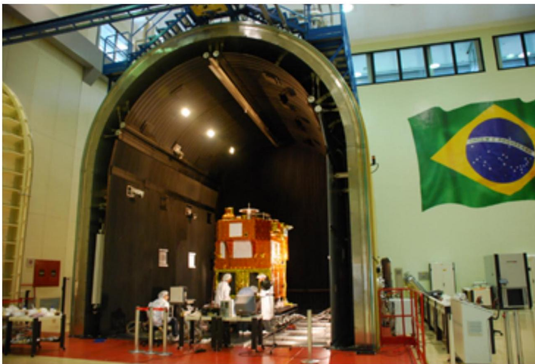
Figura 2.10: Preparação para o teste do protótipo térmico do satélite CBERS-3.
