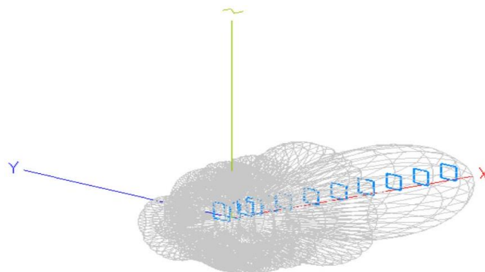
Figura 4.3: Diagrama de irradiação de uma antena direcional.
